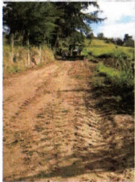
MANTENIMIENTO DE LA VIA TINA ALTA-VIA INTEROCEÁNICA
